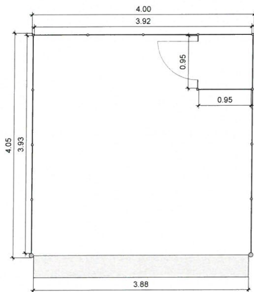
1 Planta frontis ppal. Medidas en metros
