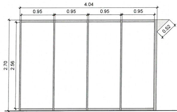
3 Alzado lateral Medidas en metros
