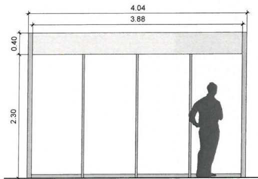
2 Alzado frontal Medidas en metros
